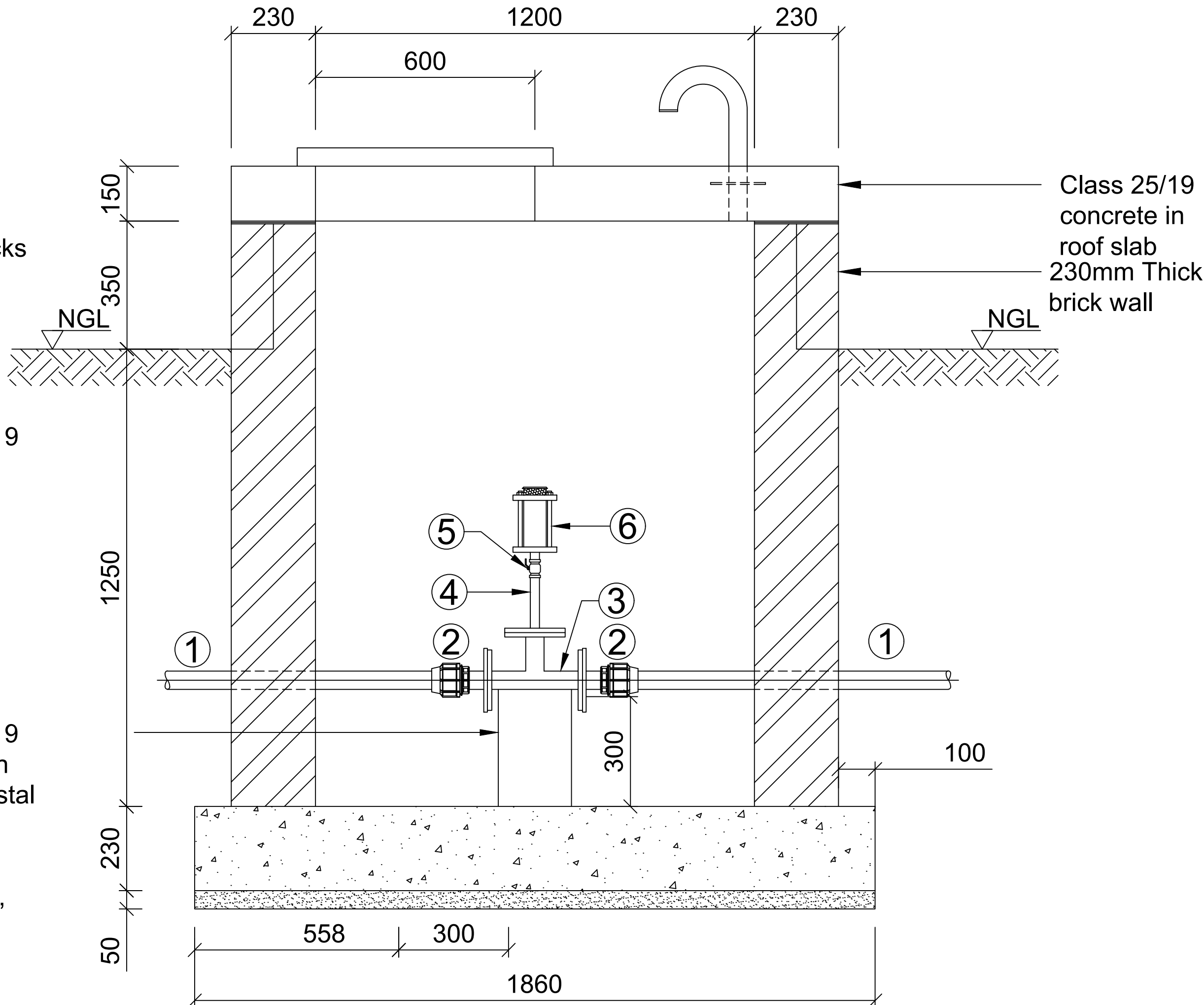
SECTION A-A 1:20
